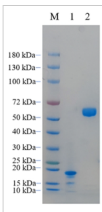
SDS-PAGE (Cat.No.: CCL25-10846H )
