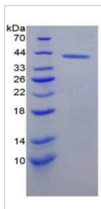
SDS-PAGE (Cat.No.: Cxcl13-79R )
